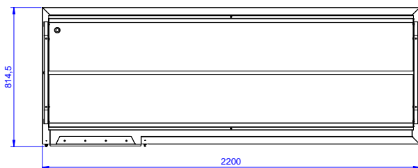
Boven aanzicht
